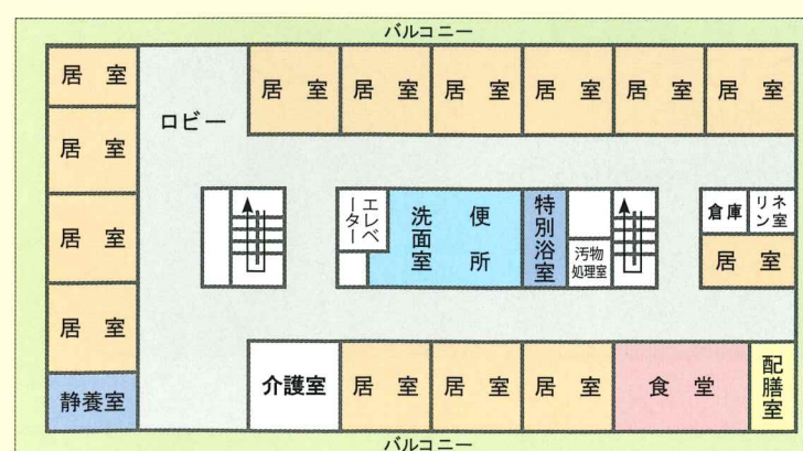
2・3階平面図
